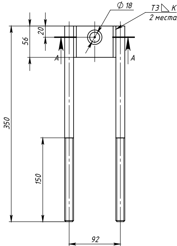
Поз.3 и Поз.4 в сборе
